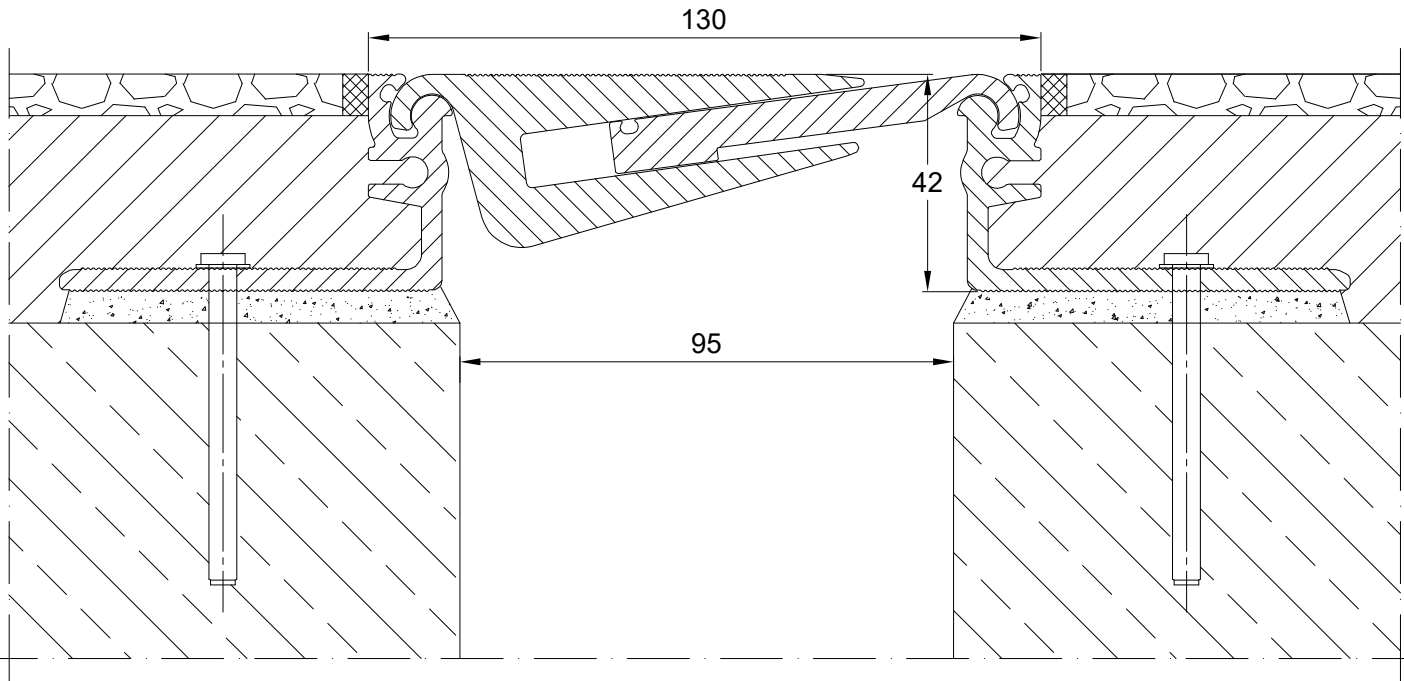
PROFIL DYLATACJNY AL 130.21.42 PRZEKRÓJ
