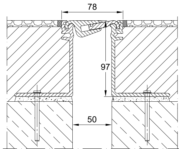
PROFIL DYLATACJNY AL 78.10.97 PRZEKRÓJ SKALA 1:2
