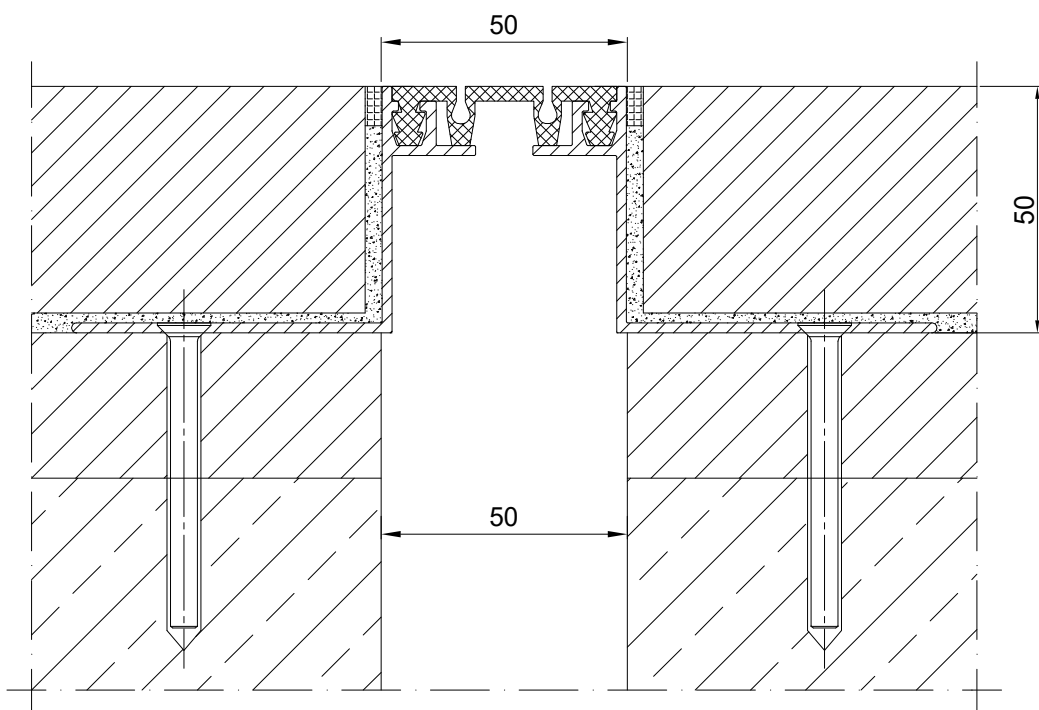
PROFIL DYLATACJNY EL 50.8.50 PRZEKRÓJ
