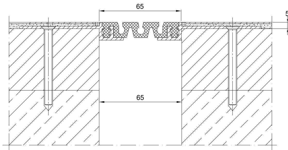
PROFIL DYLATACYJNY EL 65.10.5 PRZEKRÓJ
