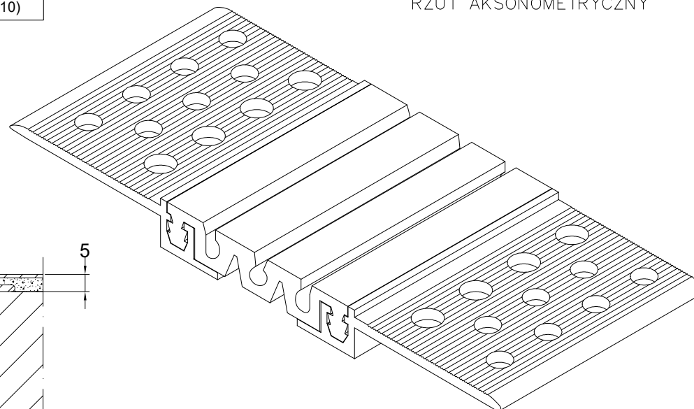
PROFIL DYLATACYJNY EL 65.10.5 RZUT AKSONOMETRYCZNY
