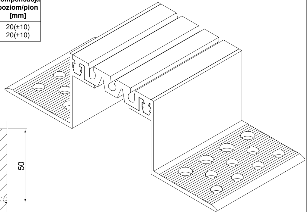
PROFIL DYLATACJNY EL 65.10.50 RZUT AKSONOMETRYCZNY
