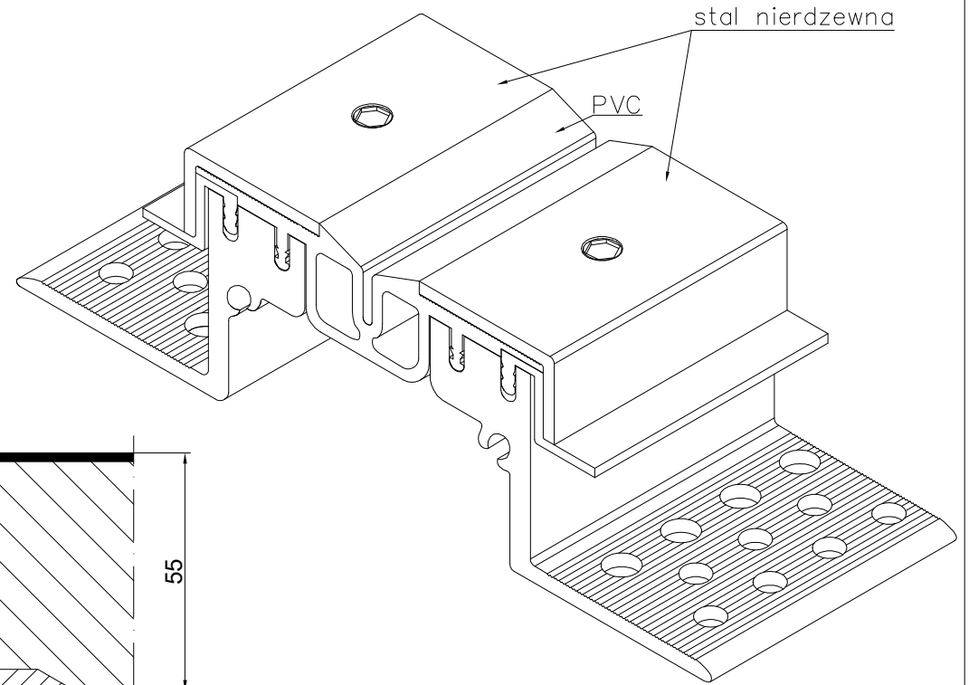
PROFIL DYLATACJNY GA 50.20.55 S RZUT AKSONOMETRYCZNY
