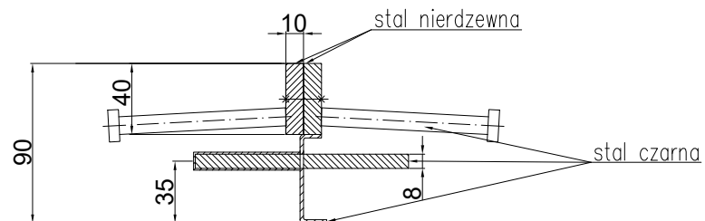
CONECTO DOWEL 10NA40-5D-T8 h=90 Przekrój
