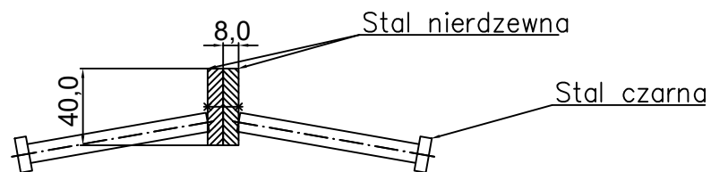
DOUBLE STRIP JOINT 08NA40 zbrojony Przekrój
