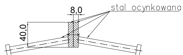
DOUBLE STRIP JOINT 08NA40 zbrojony Przekrój
