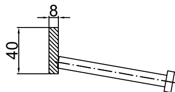
Conecto Single Strip Joint 08NA40 Przekrój
