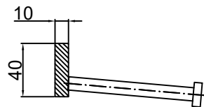
Conecto Single Strip Joint 10NA40 Przekrój
