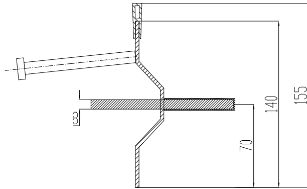
Conecto Omega 03NB-5D-T8 h=140/155 Section scale 2:1
