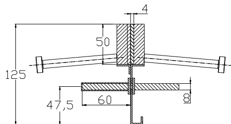
CONECTO SINUS 04NS50-4D-T8 h=125 Przekrój
