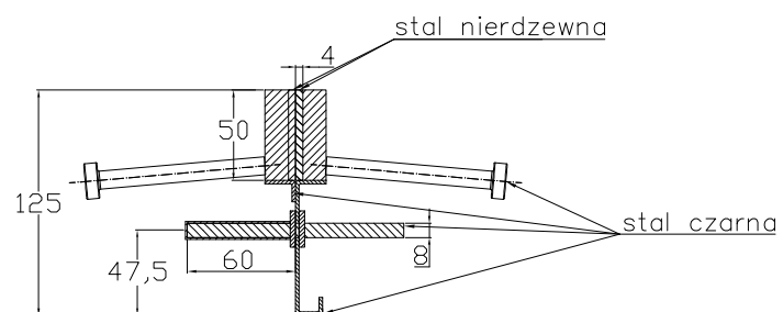
CONECTO SINUS 04NS50-4D-T8 h=125 Przekrój
