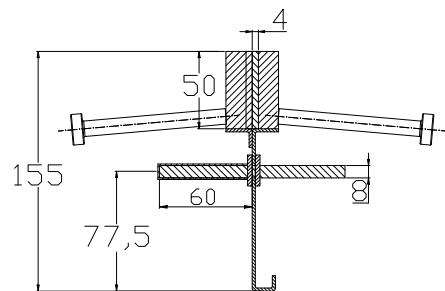
CONECTO SINUS 04NS50-4D-T8 h=155 Przekrój
