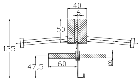
CONECTO SINUS 06NS50-4D-T8 h=125 Przekrój
