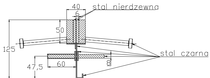
CONECTO SINUS 06NS50-4D-T8 h=125 Przekrój
