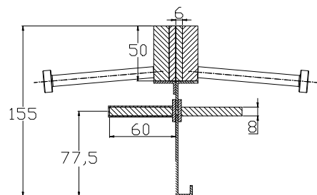
CONECTO SINUS 06NS50-4D-T8 h=155 Przekrój
