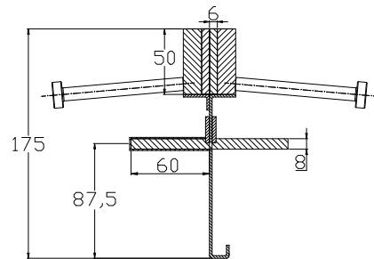
CONECTO SINUS 06NS50-4D-T8 h=175 Przekrój
